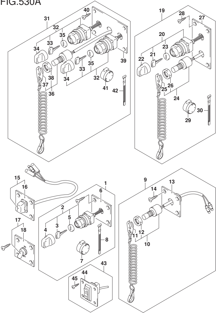
DF140A_E11_019_530A OPT:SWITCH
