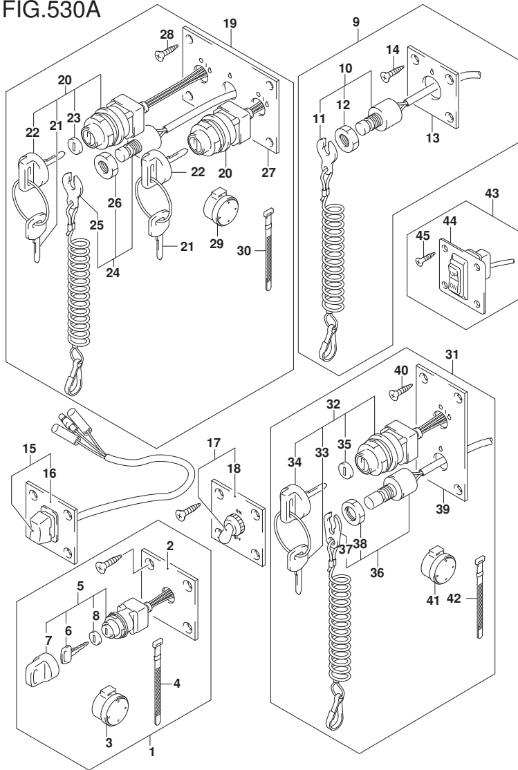
FIG.530A (1-J-3) OPT:SWITCH
