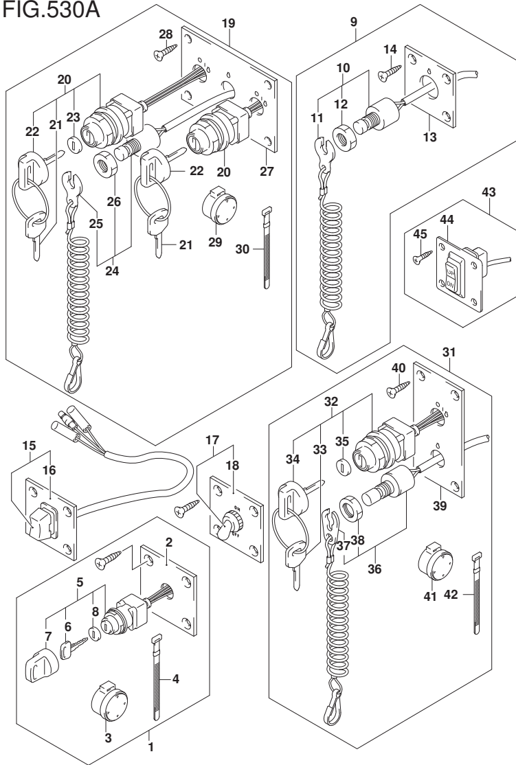
FIG.530A (1-J-2) OPT:SWITCH
