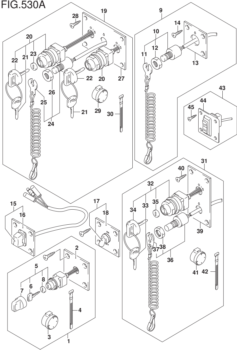
FIG.530A (1-J-4) OPT:SWITCH
