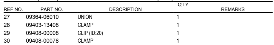
FIG.143B (1-C-9) FUEL VAPOR SEPARATOR (E40)
