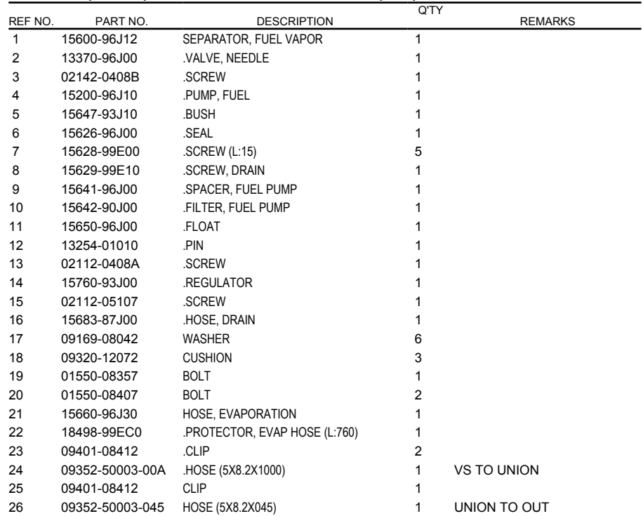
FIG.143B (1-B-15) FUEL VAPOR SEPARATOR (E40)
