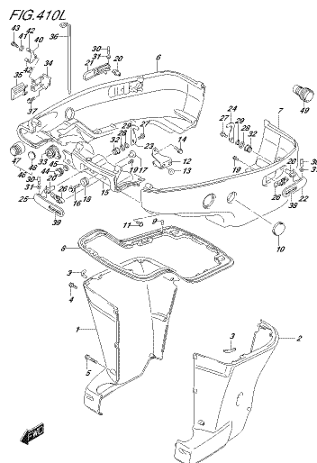
FIG. 410L DSC90 REV. 015, 410L DSE 00862
