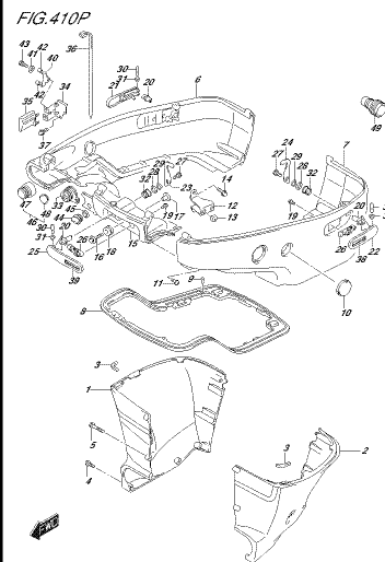
FIG. 410P DSC90 REV. 015, 410P DSE 00862
