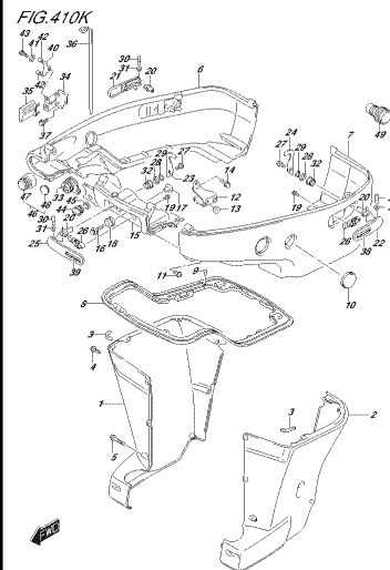
FIG. 410K DSC90 REV. 015, 410K DSE 00862
