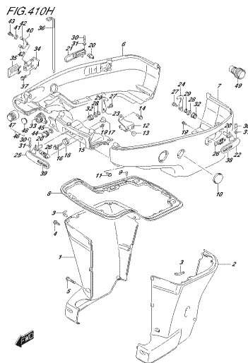
FIG. 410H DSC90 REV. 015, 410H DSE 00862
