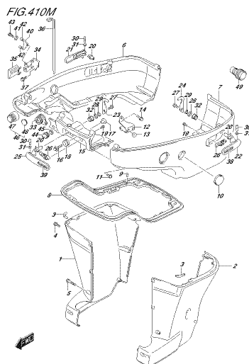
FIG. 410M DSC90 REV. 015, 410M DSE 00862
