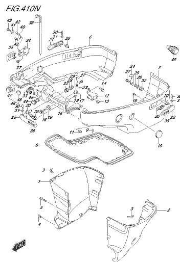
FIG. 410N DSC90 REV. 015, 410N DSE 00862
