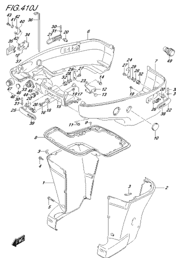
FIG. 410J DSC90 REV. 015, 410J DSE 00862
