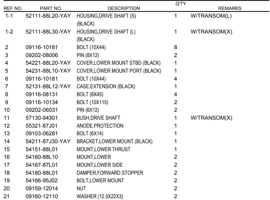
FIG.405J (1-L-14) DRIVE SHAFT HOUSING (DF60AVT:E01,DF60AVT:E40)
