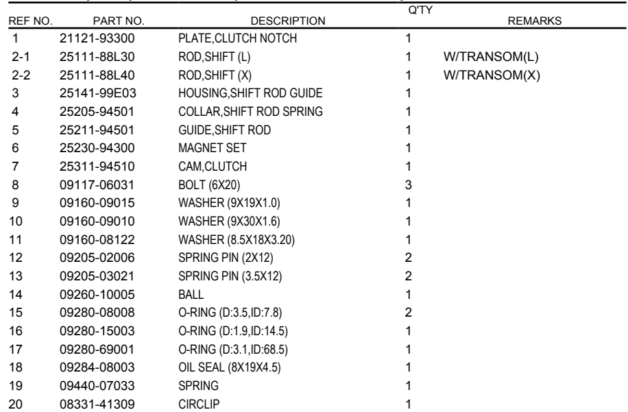
FIG.210B (1-F-3) SHIFT ROD (DF60AVT,DF60AVTH)
