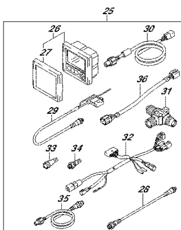
FIG.503A (4-I-6) OPT:METER (2)
