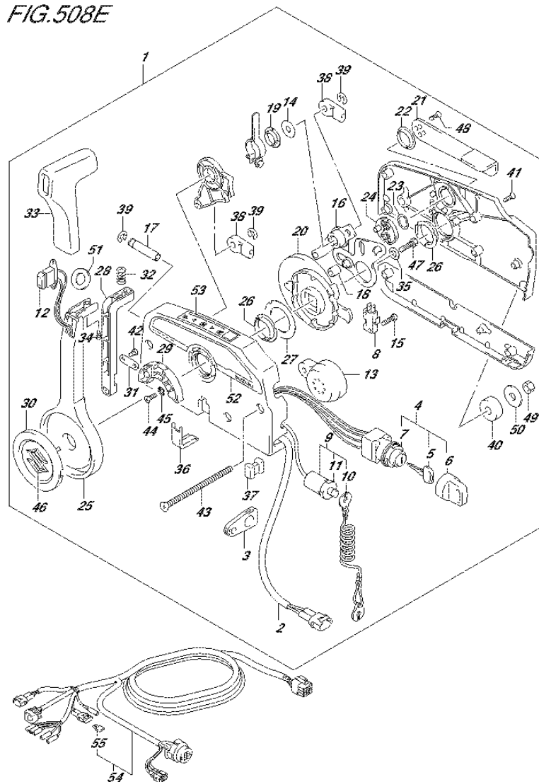
FIG.508E (3-C-4) OPT:REMOTE CONTROL (DF80A E40)
