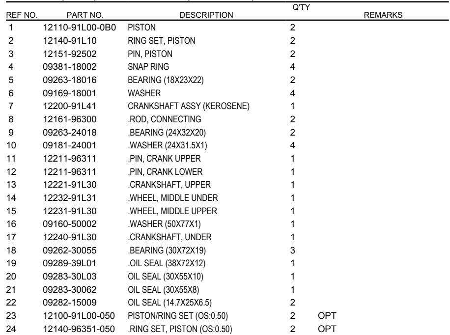
FIG.116A (1-B-5) CRANKSHAFT (DT25K P36)
