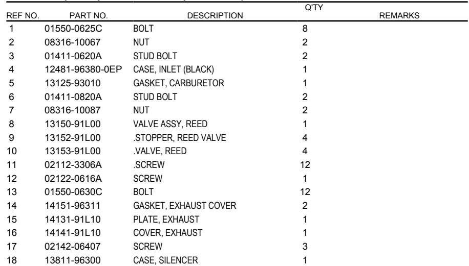
FIG.125B (1-B-9) INLET CASE (DT30 P40)
