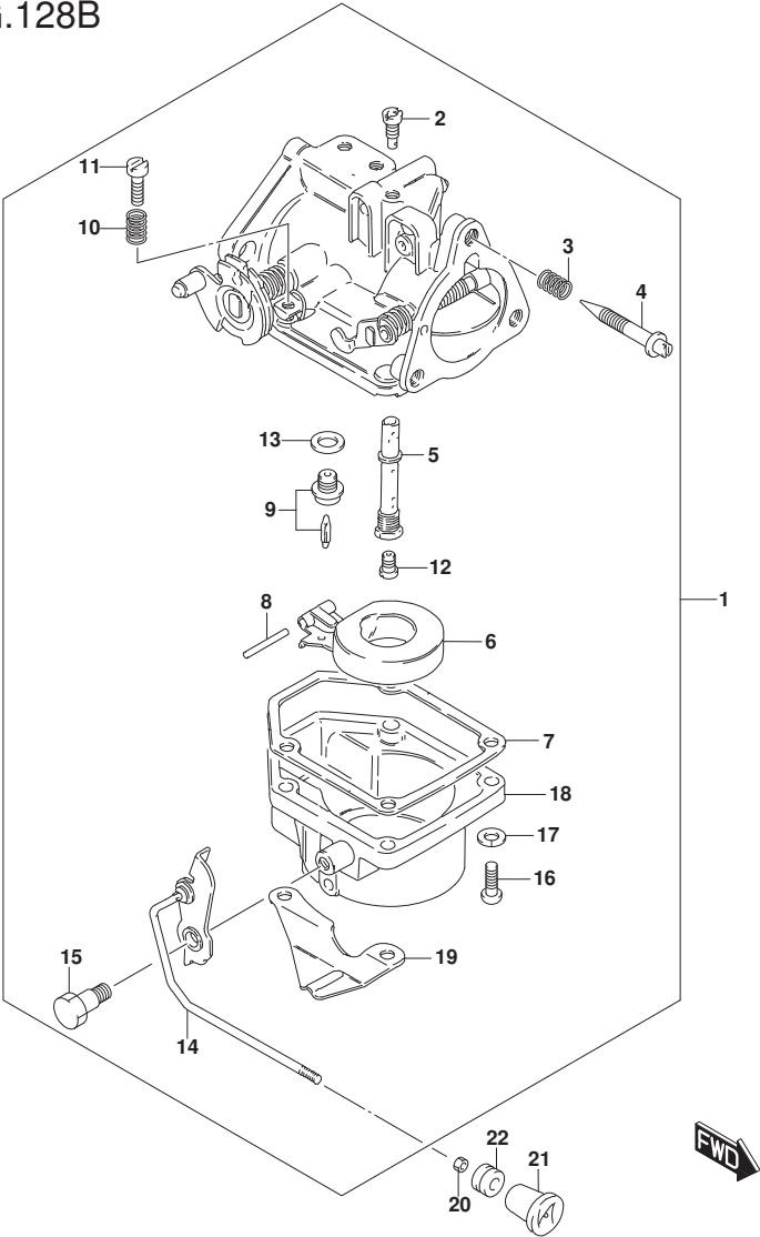
FIG.128B (1-B-10) CARBURETOR (DT30)(DT30R)
