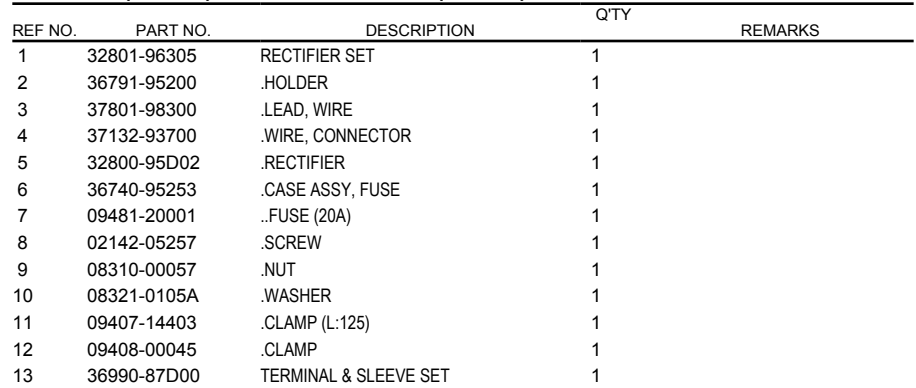
FIG.550A (1-G-11) OPT:ELECTRICAL (DT25K)
