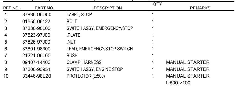
FIG.319E (1-G-5) ELECTRICAL (DT15AK P36)
