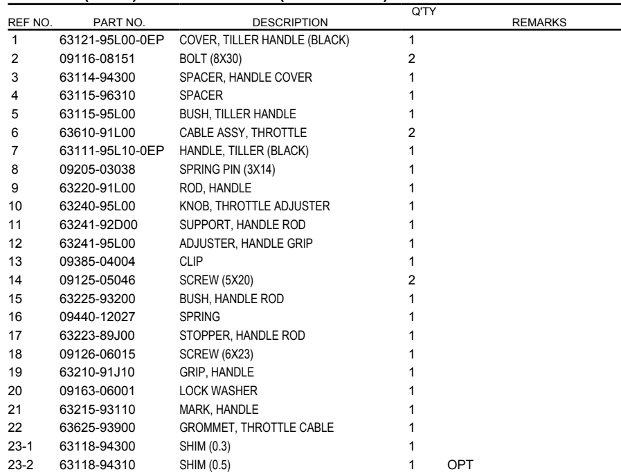
FIG.444E (1-I-12) TILLER HANDLE (DT15AK P36)
