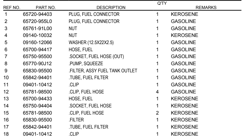
FIG.430A (1-G-8) FUEL HOSE (DT9.9AK P36)(DT15AK P36)
