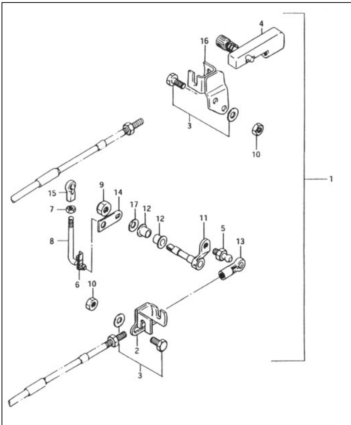
FIG.50 SISTEMA DE DIREÇÃO OPCIONAL
